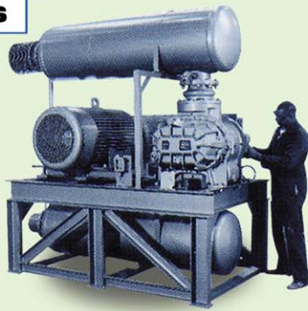
รูทโบลเวอร์และแวกคัมปั้ม (Roots Blower, Vacuum Pump)
